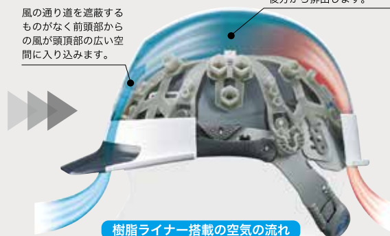
樹脂ライナー搭載の空気の流れ
